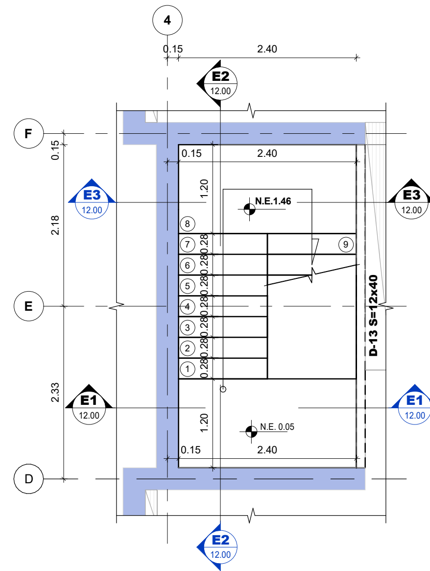
PLANTA ARRANQUE ESCALERA TIPO 1 (PISO 1 A 2) Escala 1 : 50
