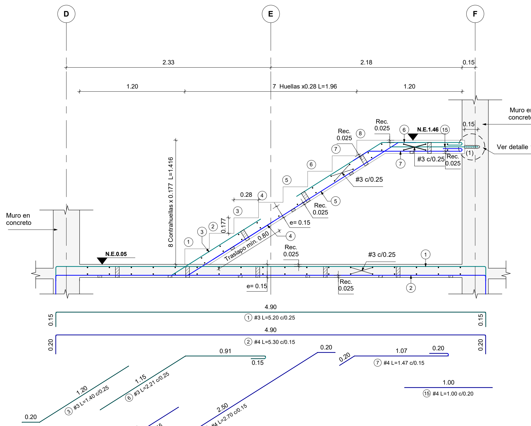
CORTE E-2 Escala 1 : 25
