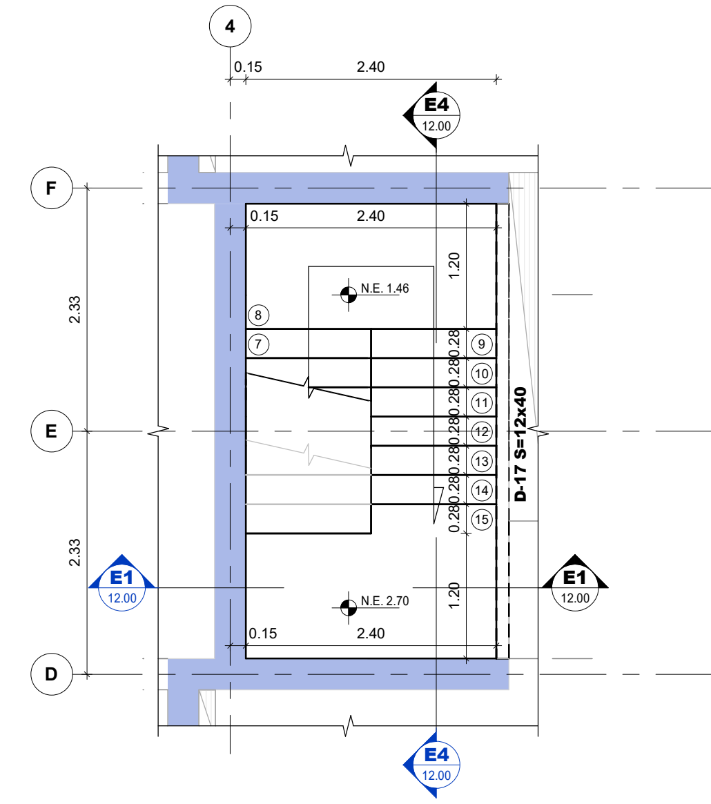
PLANTA LLEGADA ESCALERA TIPO 1 (PISO 1 A 2) Escala 1 : 50
