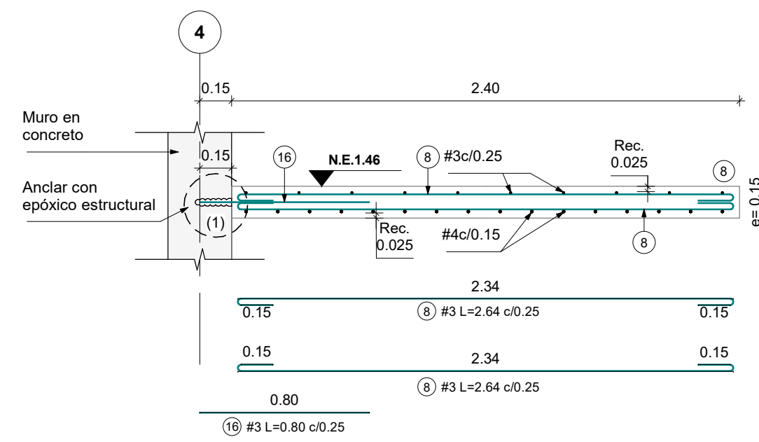
CORTE E-3 Escala 1 : 25
